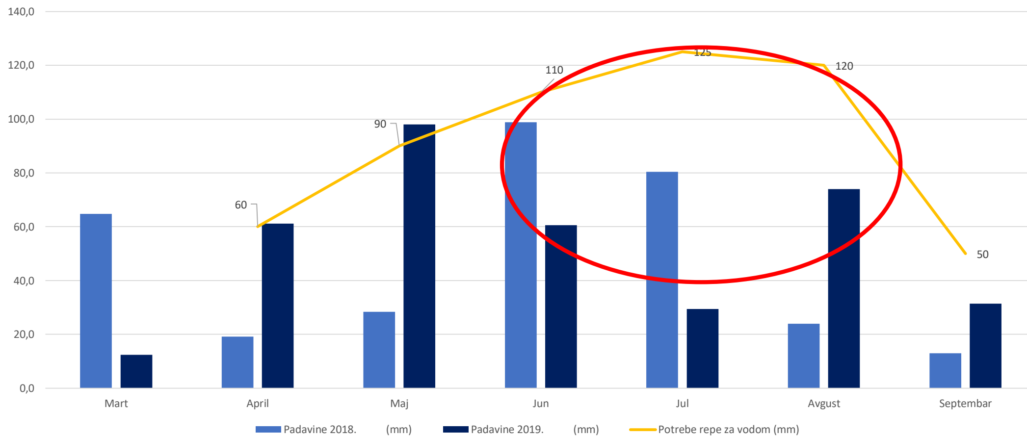
Vrbas padavine (mm) u periodu vegetacije 2018/2019.
